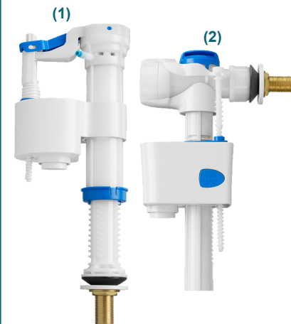
MECANISMO UNIVERSAL ROCA DESCARGA DOBLE
